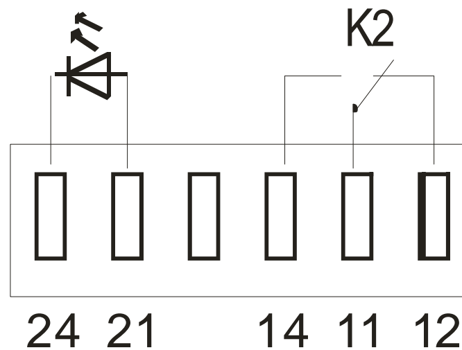
Abbildung 4: Klemmenbelegung
