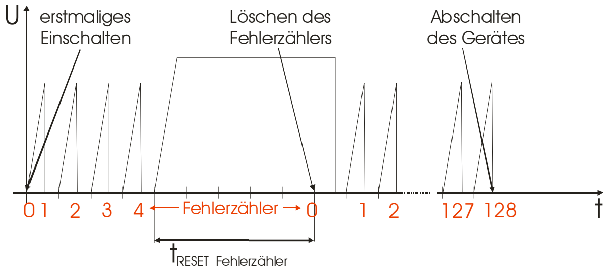
Abbildung 2: Löschen des Fehlerzählers / Geräteabschaltung
