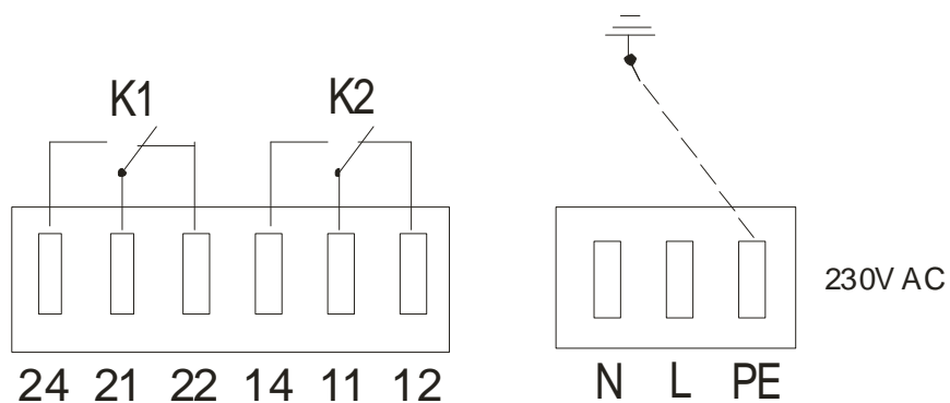
Abbildung 4: Klemmenbelegung
